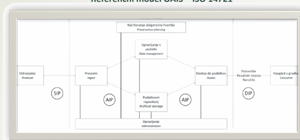
Referenčni model OAIS – ISO 14721
